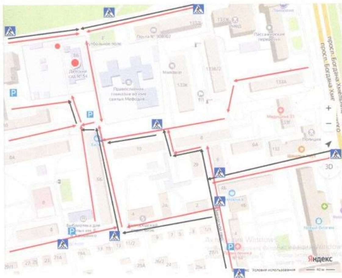
2.2. Схема организации дорожного движения в непосредственной близости от дошкольной образовательной организации с размещением соответствующих технических средств организации дорожного движения детей и расположением парковочных мест.
